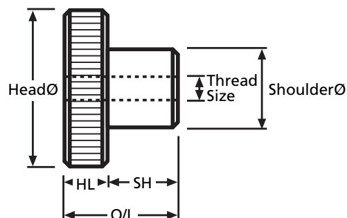
PTN Type
